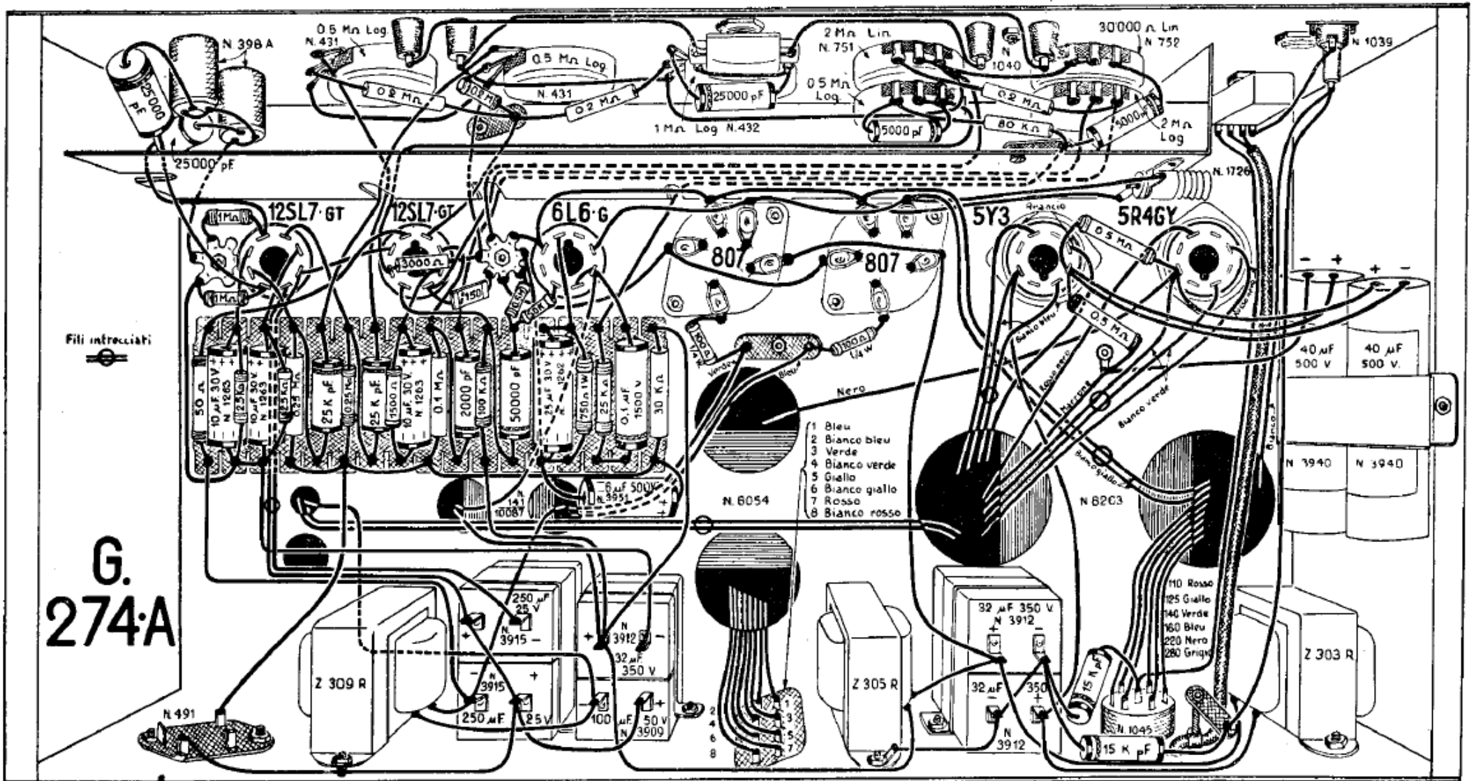
Lo schema di montaggio.
